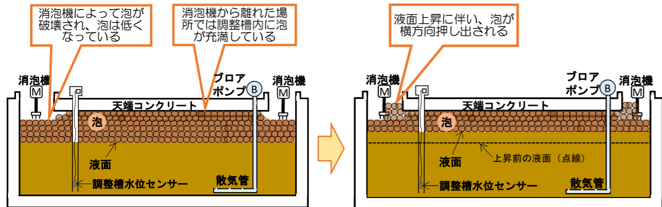
図-3 調整槽内部の断面図
