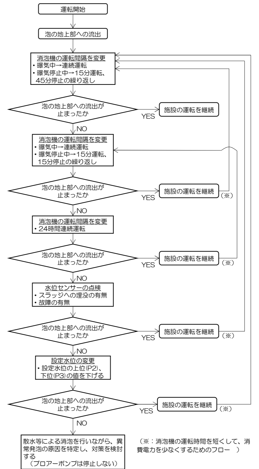
図-5 泡流出時の対処フロー
